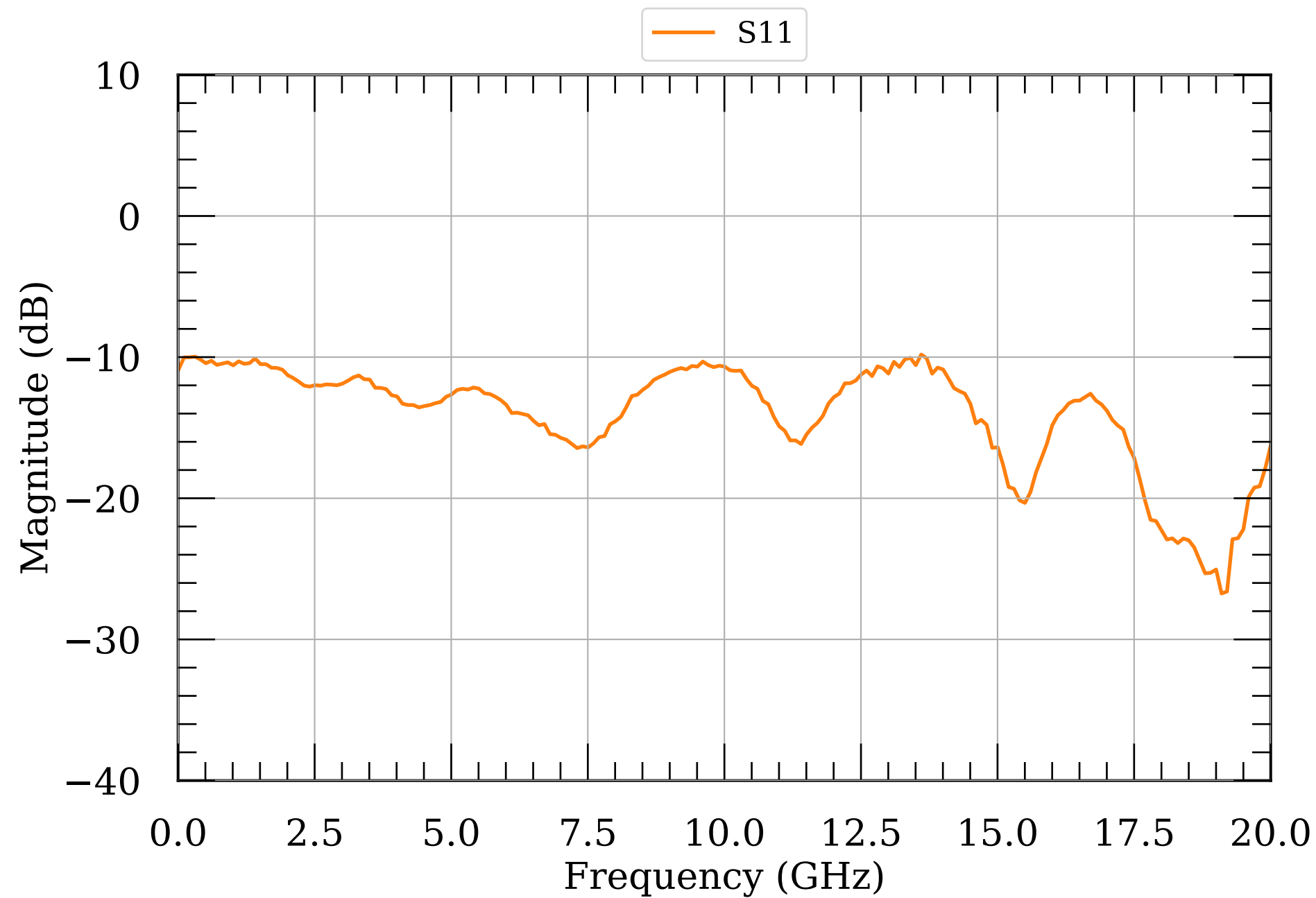
LNA S-params module055
